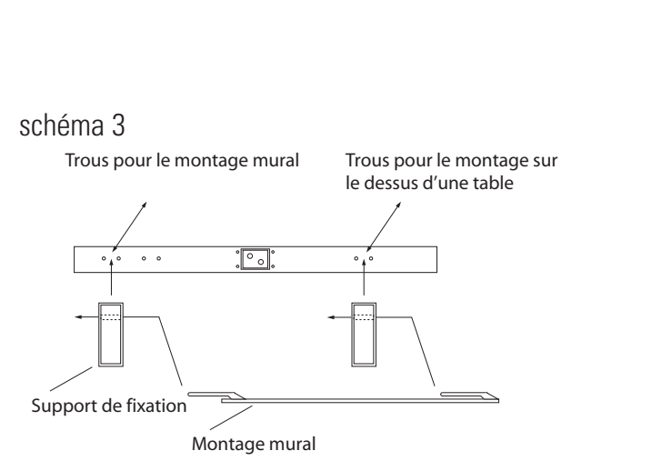
schéma 3
