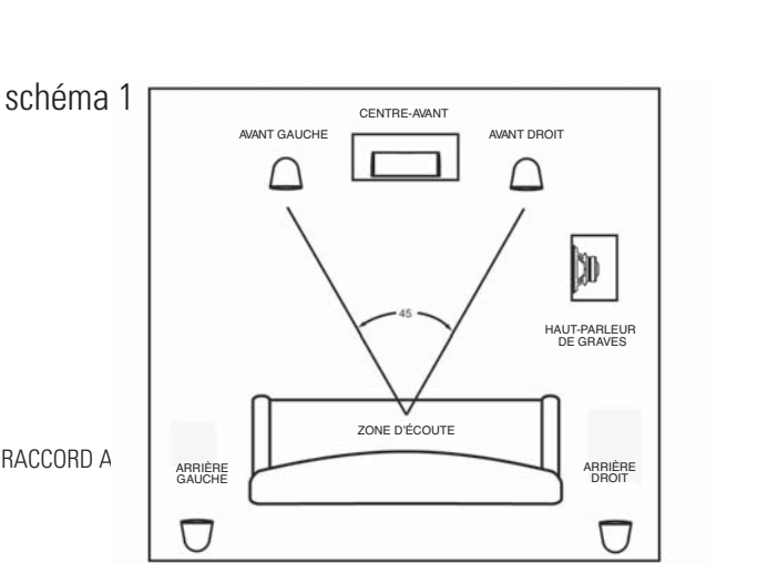
schéma 1
